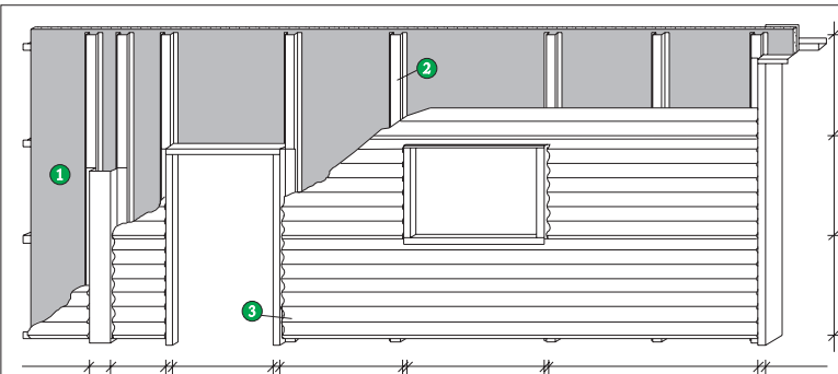
Fasado brėžinys
