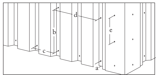
Tvirtinimo sraigtų sukimo vietos montuojant vertikaliai
