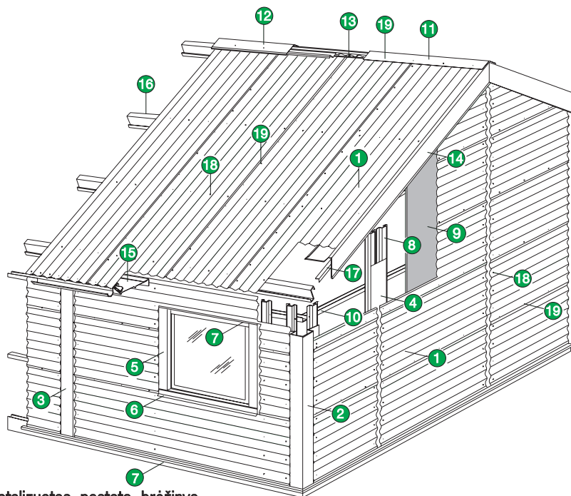
Detalizuotas pastato brėžinys
